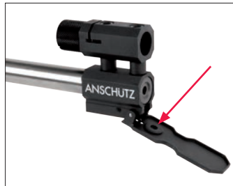
Gummipfropfen bei versehentlichem Auslösen mit verschlossener Schneeklappe. Rubber plug in case of inadvertent shot release at closed snow cover. Best.-Nr.: 004252
