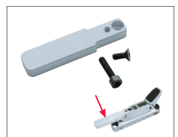
Kappenverlängerung für 4759 , für Aufлагeschießen. Butt plate extension, for 4759 , for benchrest shooting. Best.-Nr.: 008432
